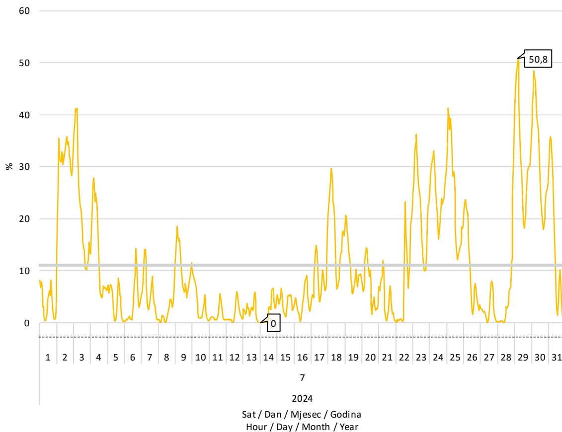
Slika 8 Udio proizvodnje vjetroelektrana u pokrivanju satnog opterećenja elektroenergetskog sustava u srpnju 2024. godine
