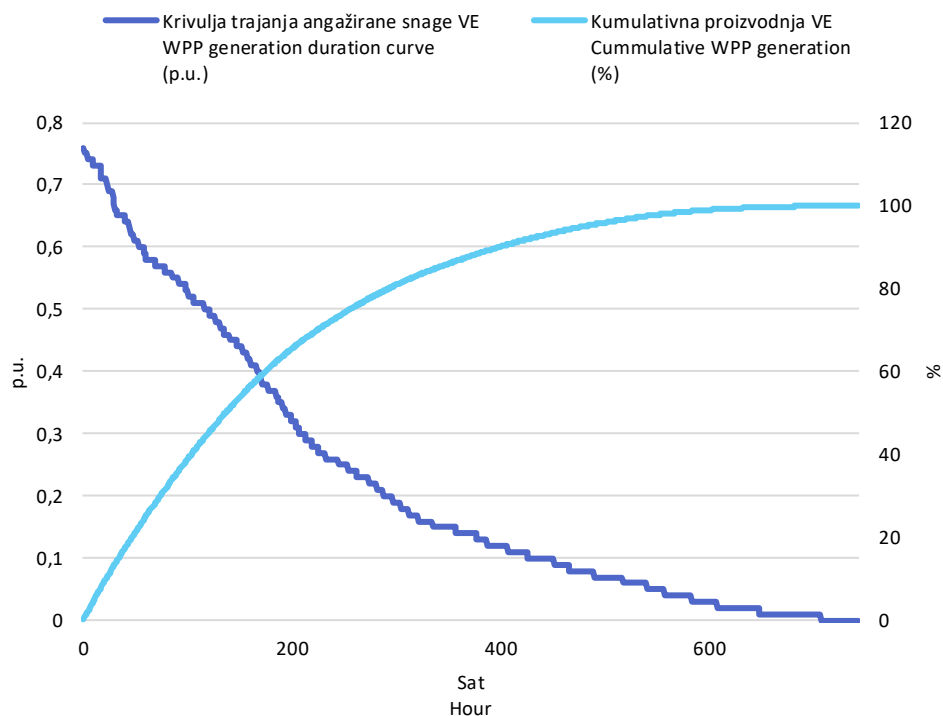
Slika 3 Krivulja trajanja angažirane snage svih VE i kumulativna proizvodnja VE u srpnju 2024. godine u jediničnim vrijednostima
