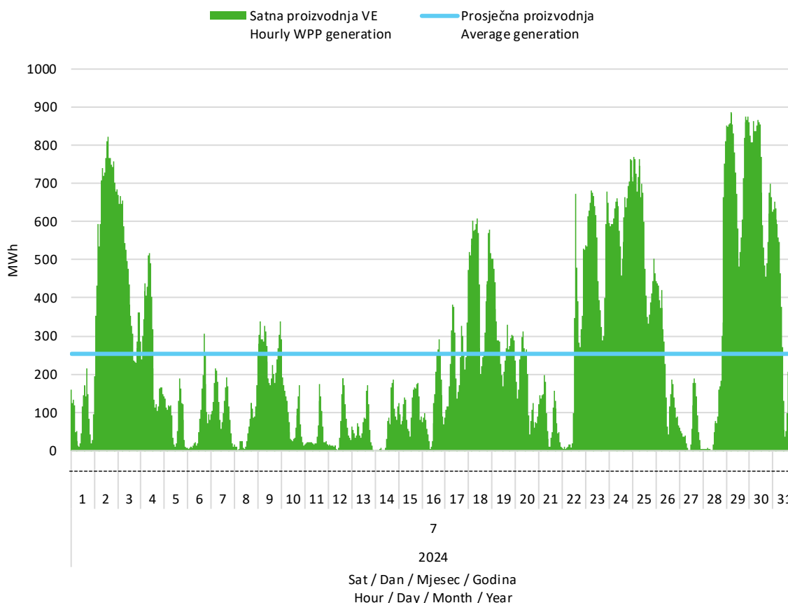
Slika 2 Satna proizvodnja svih vjetroelektrana u srpnju 2024. godine
