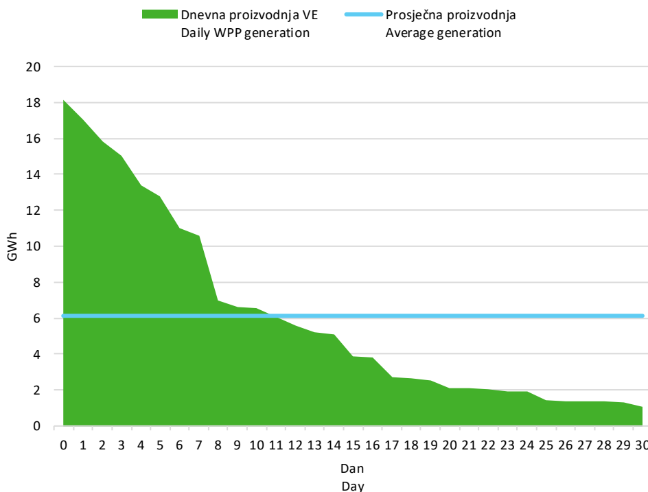
Slika 6 Krivulja trajanja dnevne proizvodnje vjetroelektrana u srpnju 2024. godine
