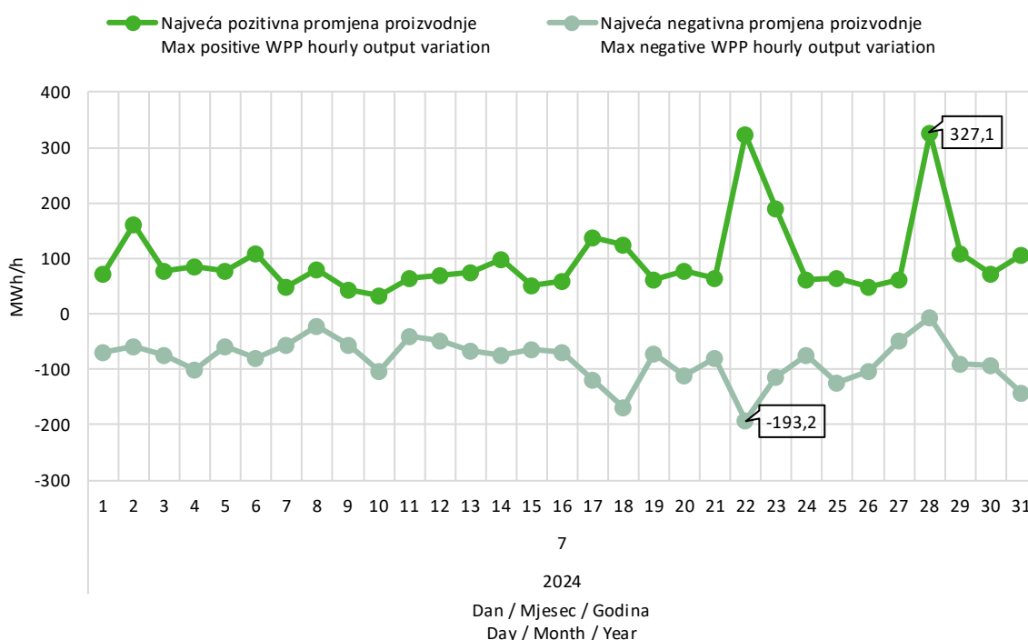
Slika 9 Maksimalna pozitivna i maksimalna negativna promjena satne proizvodnje VE u srpnju 2024. godine
