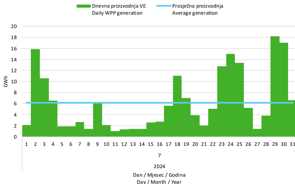
Slika 5 Dnevna proizvodnja svih vjetroelektrana u srpnju 2024. godine
