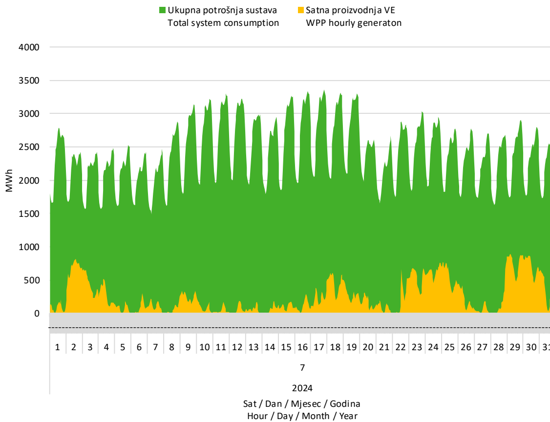
Slika 7 Usporedba satnog dijagrama opterećenja sustava i proizvodnje vjetroelektrana u srpnju 2024. godine
