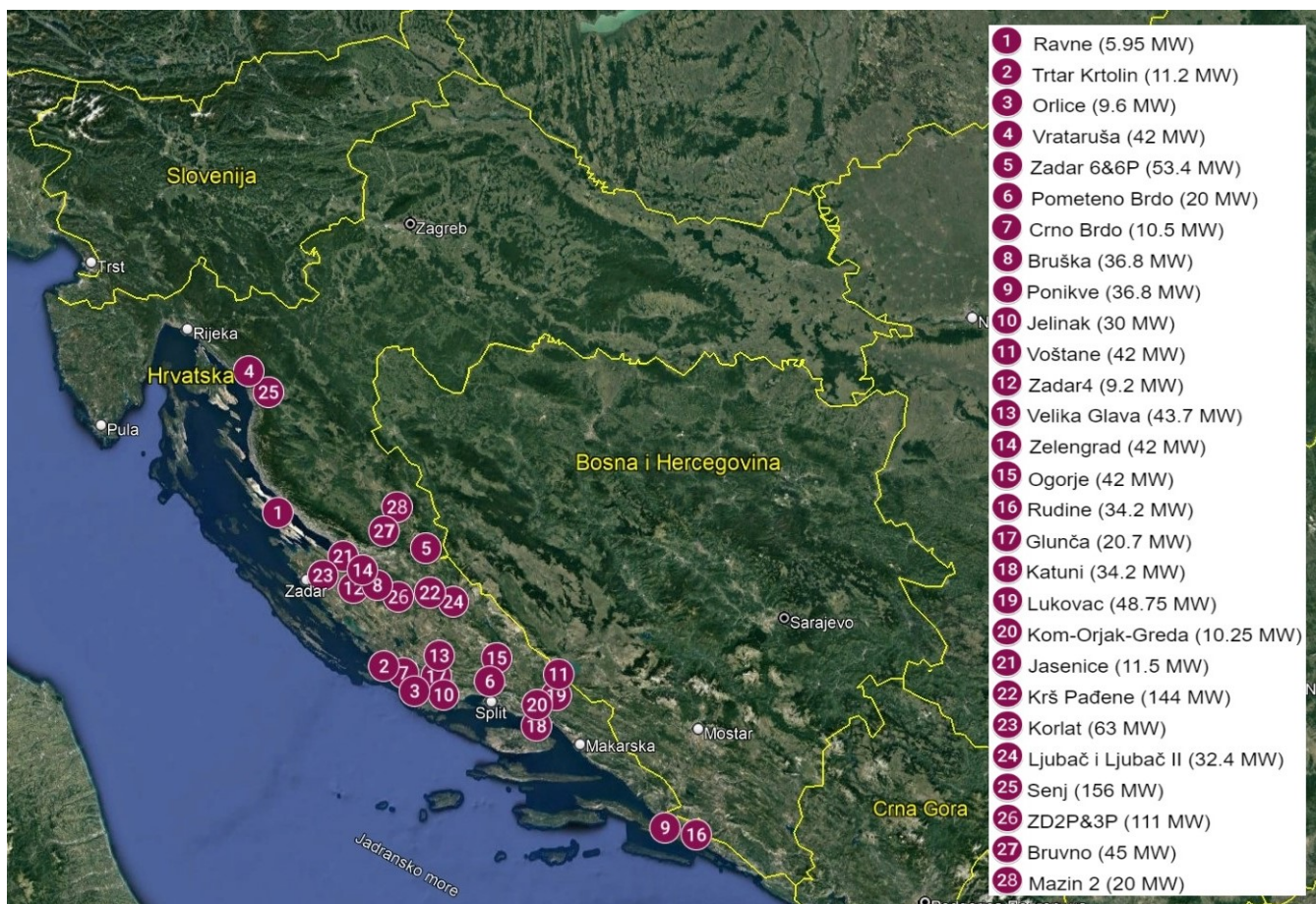
Slika 1 Lokacije VE u Hrvatskoj Figure 1 WPP locations in Croatia
